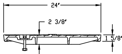
LID SECTION B-B
